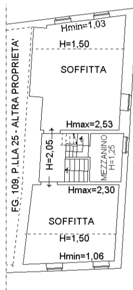
PIANO TERZO
