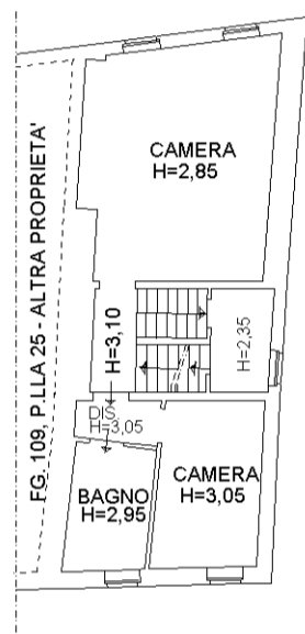
PIANO SECONDO
